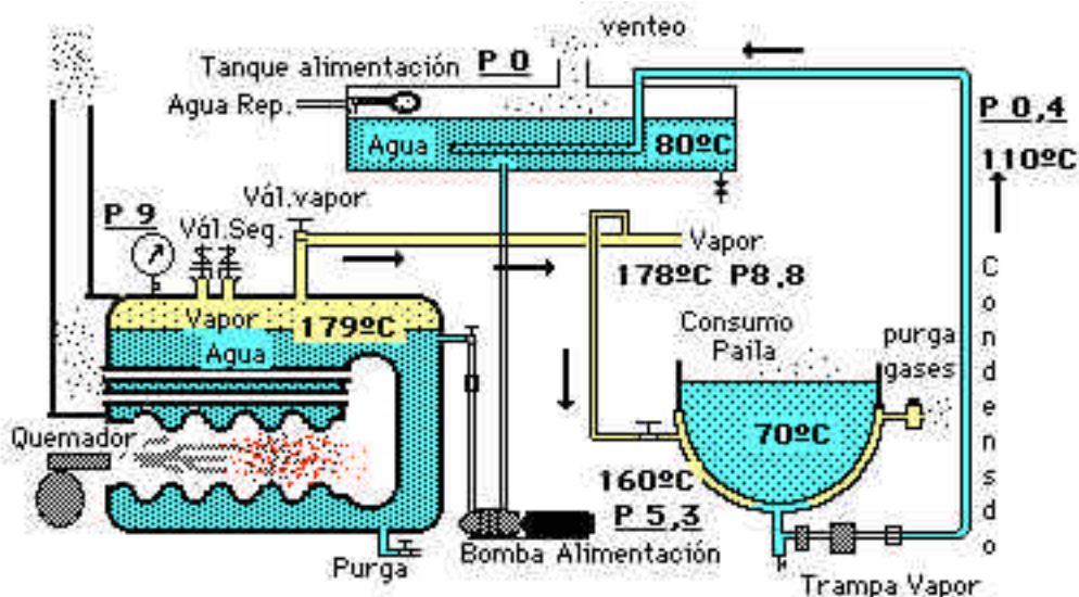
El ciclo del agua y el vapor transportando calor P = \text{Kgr/cm}^2 \text{ (Rel.)}
