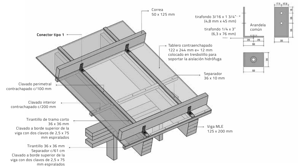
FIGURA 2. CUBIERTA CON VIGAS DE MADERA LAMINADA ENCOLADA. FUENTE: DOCUMENTO COMENTADO EN EL ARTÍCULO
