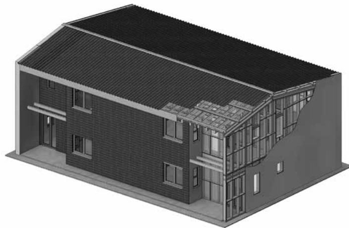
FIGURA 1. PROTOTIPO DE VIVIENDA DE DOS NIVELES CON ESTRUCTURA DE ENTRAMADO LIGERO DE MADERA. FUENTE: DOCUMENTO COMENTADO EN EL ARTÍCULO
