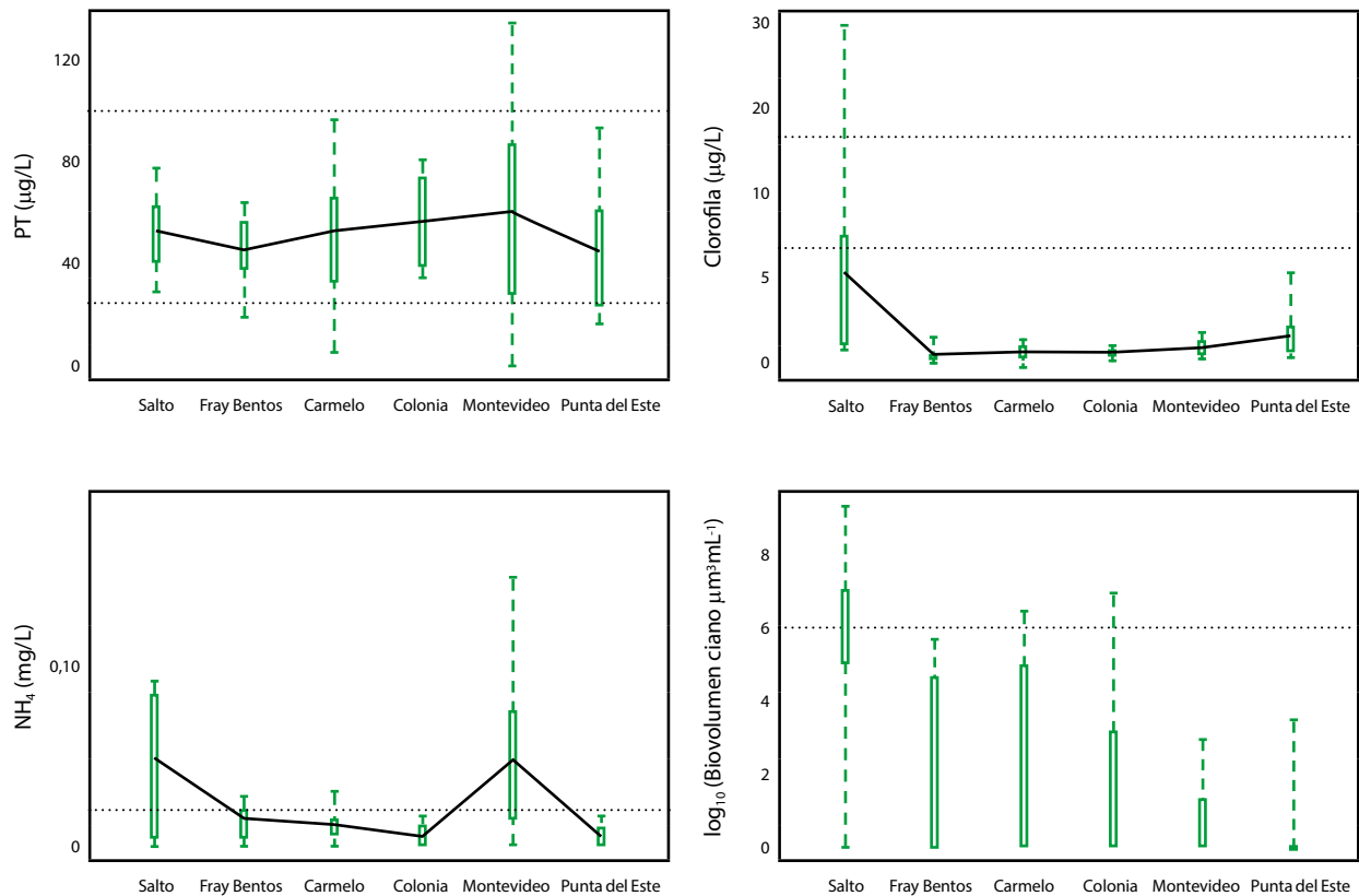
Figura 3. Variación espacial de la concentración de fósforo total (PT), amonio ( \text{NH}_4 ) y biovolumen total de cianobacterias.
